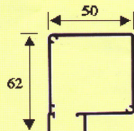
CASSONETTO 50 mm
