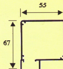
CASSONETTO 55 mm
