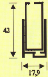
GUIDA TELESCOPICA
